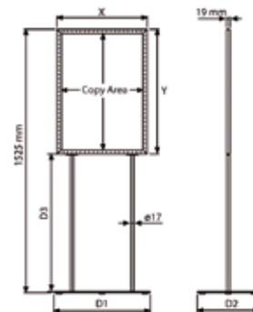
H-Fuß Plakatständer optional H-Feet Info Board optional
